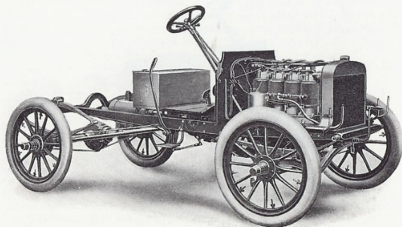
FORD MODEL B, CHASSIS.
