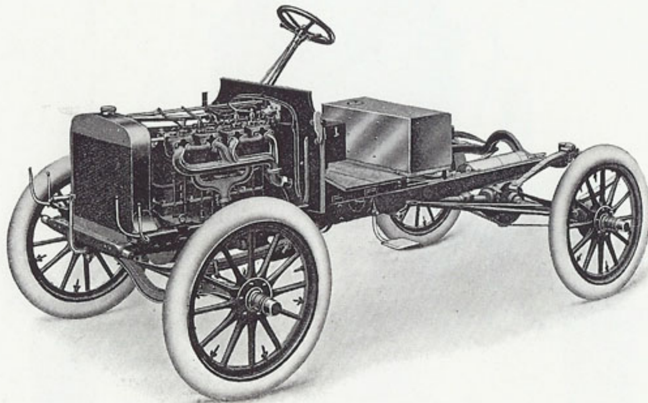
FORD MODEL B, CHASSIS.
